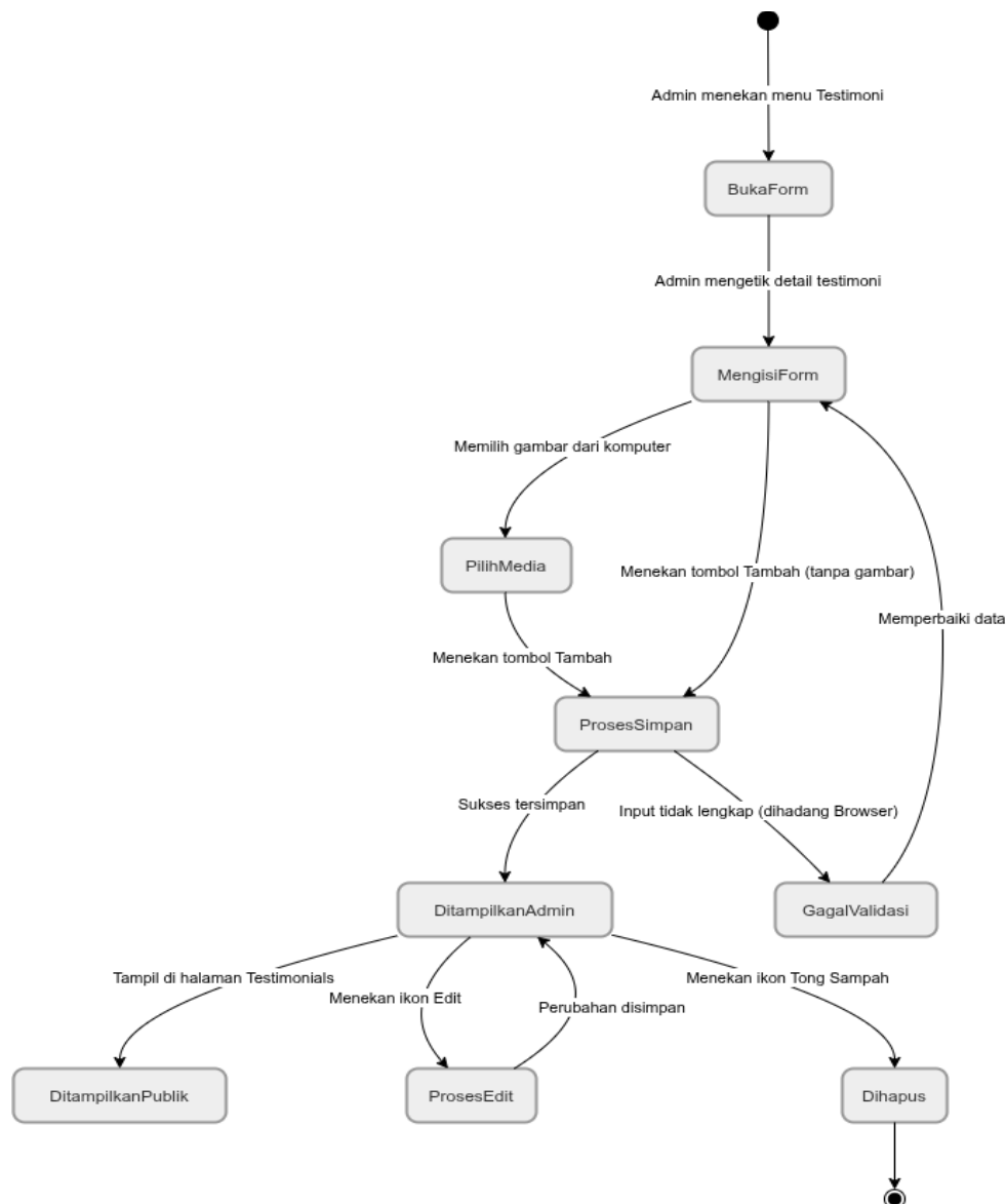
Gambar 1. Alur penggunaan menggunakan flowchart
